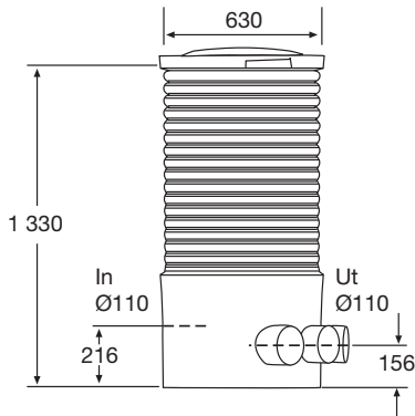
Fördelningsbrunn
