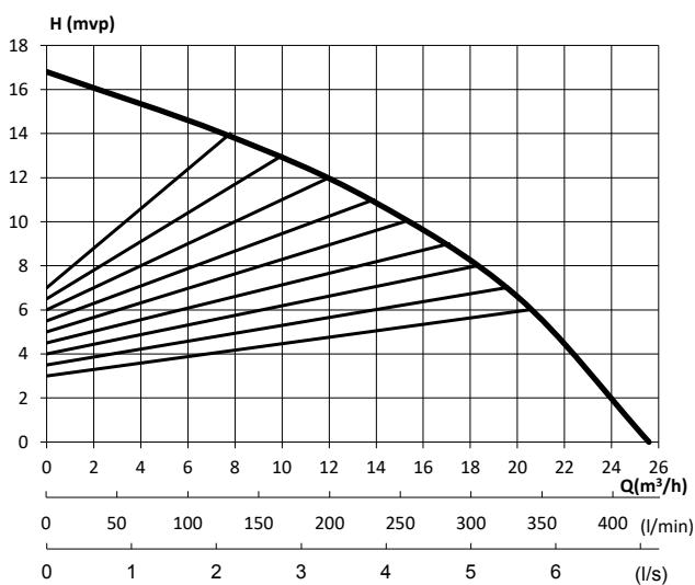
Kapacitetsdiagram (D)40-16/26
