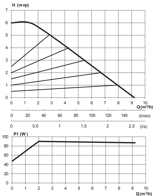
Kapacitetsdiagram 25U & 30U -6/9
