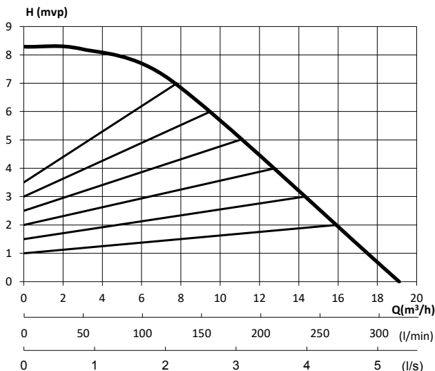
Kapacitetsdiagram (D)40-8/18
