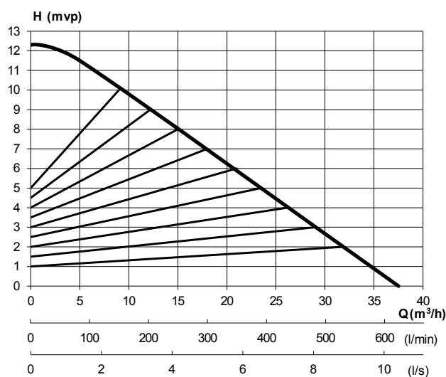
Kapacitetsdiagram(D)50-12/37
