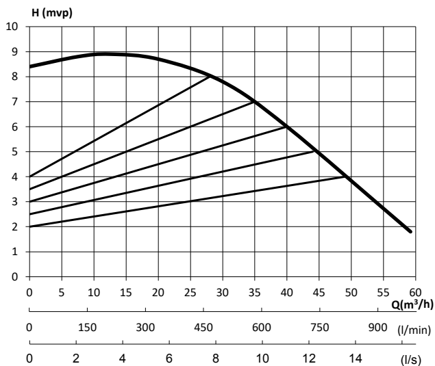
Kapacitetsdiagram 100-18/73
