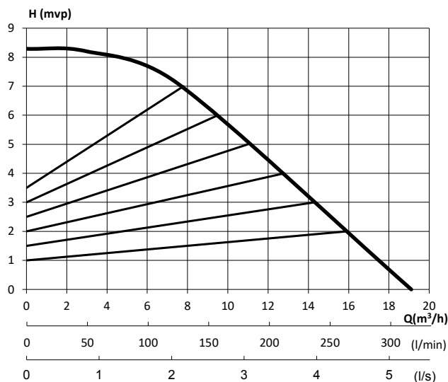
Kapacitetsdiagram (D)40-8/18
