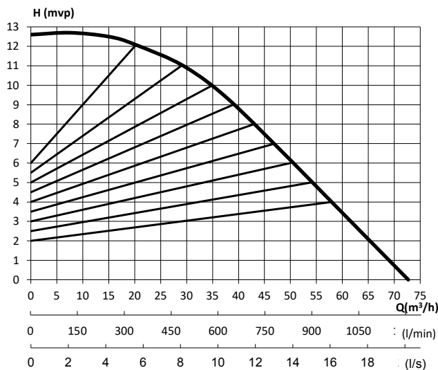
Kapacitetsdiagram 100-12/72
