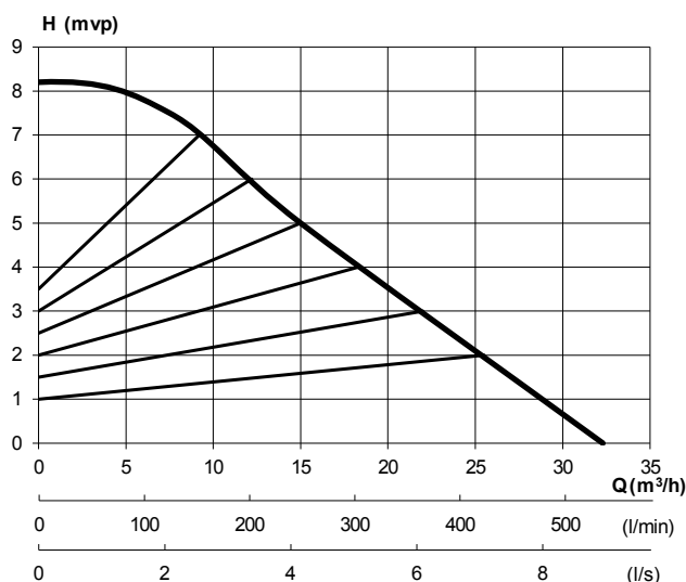
Kapacitetsdiagram(D)50-8/32
