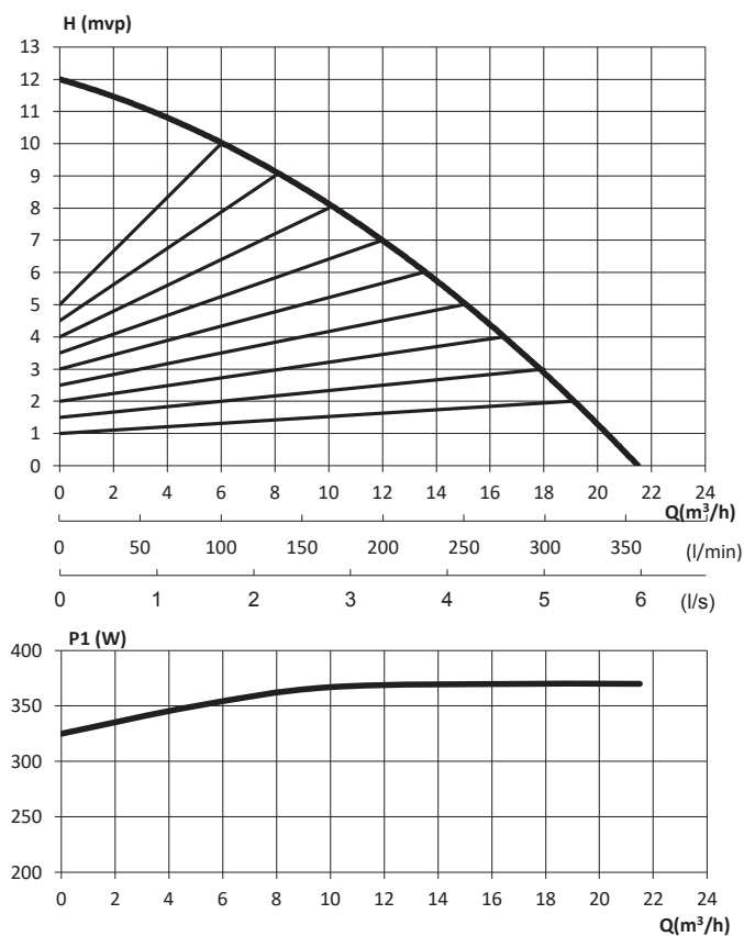
Kapacitetsdiagram 32F-12/21
