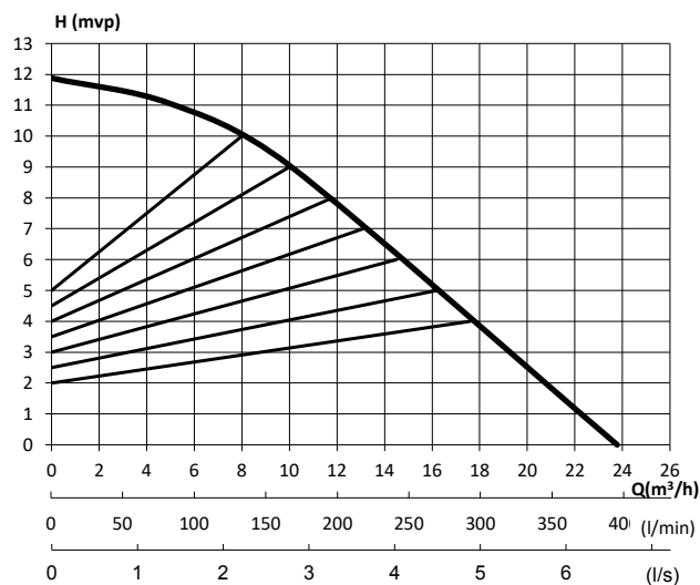
Kapacitetsdiagram (D)40-12/24
