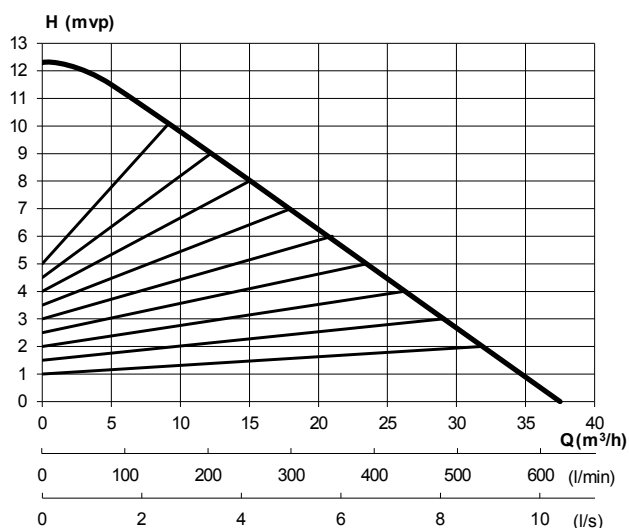
Kapacitetsdiagram(D)50-12/37
