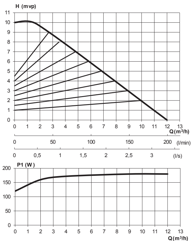
Kapacitetsdiagram 25-50 -10/12
