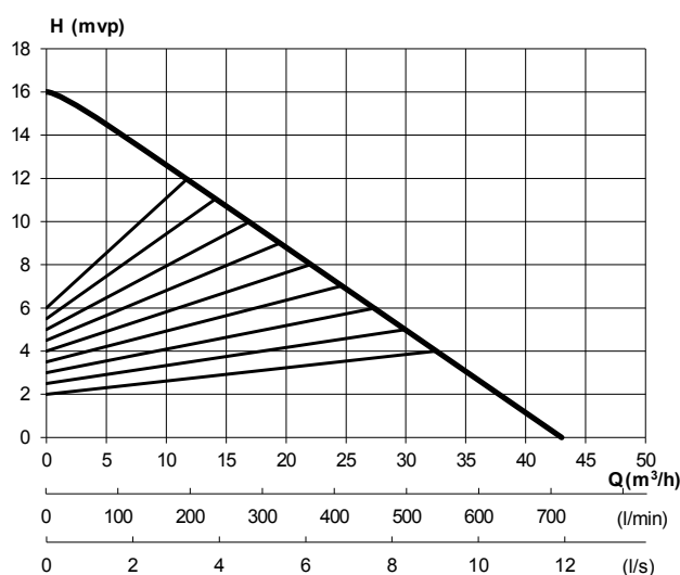
Kapacitetsdiagram ((D)50-16/43
