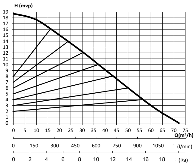
Kapacitetsdiagram 100-18/73
