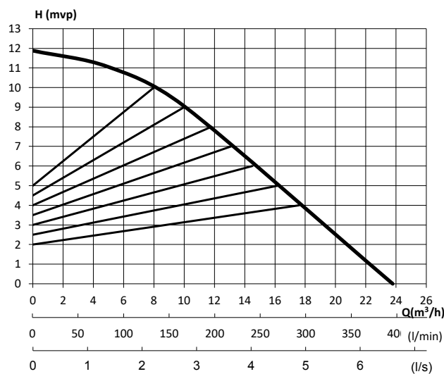
Kapacitetsdiagram (D)40-12/24
